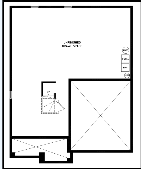
Elev A
