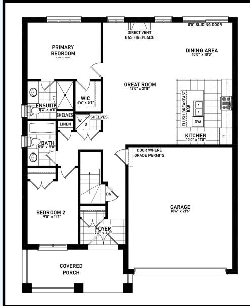
Elev B
