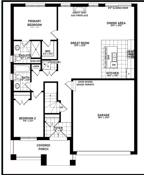
Elev A
